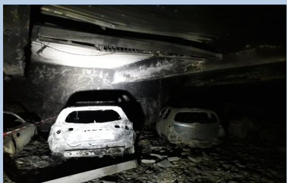
Fissuration d'origine thermique sur poutre BA (SDIS33-2019)
