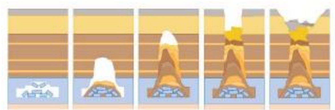
Mécanismes de remontée à la surface d'une cloche d'effondrement, dû à la dégradation du toit de la cavité
