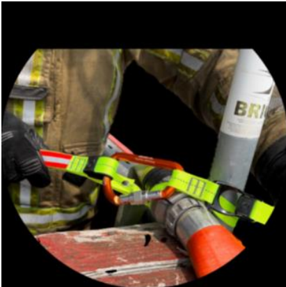
Continuer le serrage jusqu'à ce que le raccord soit bien plaqué sur le point fixe.
