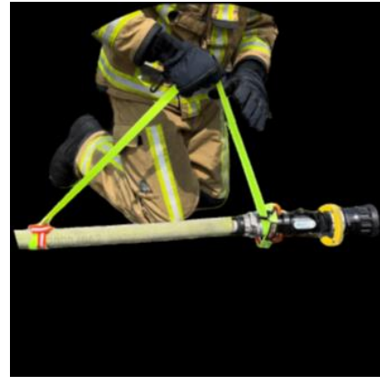
Serrer l'ensemble en vérifiant que la sangle soit bien sur le demi-raccord côté lance.
