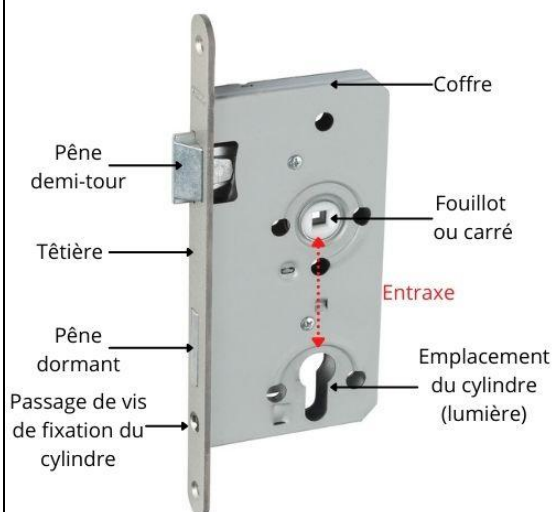
Serrure à encastrer
