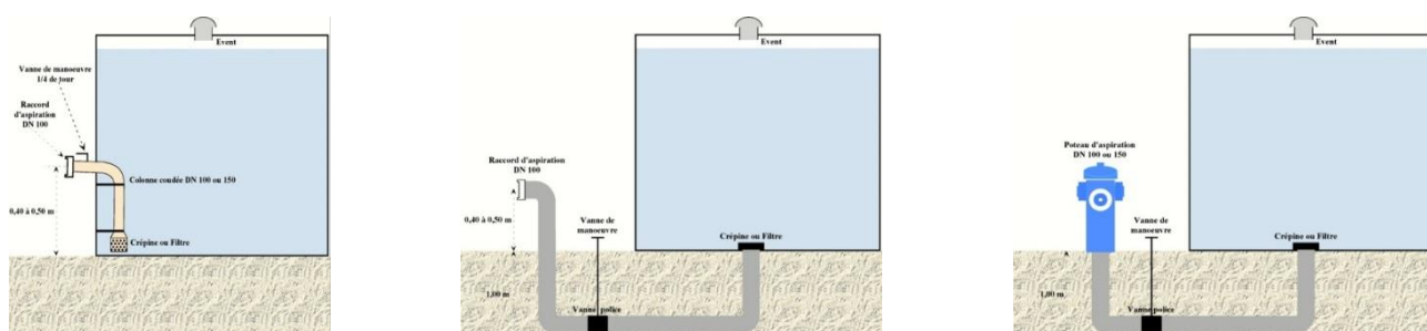
Illustration n°11: Différents dispositifs d'aspiration sur réservoir aérien
