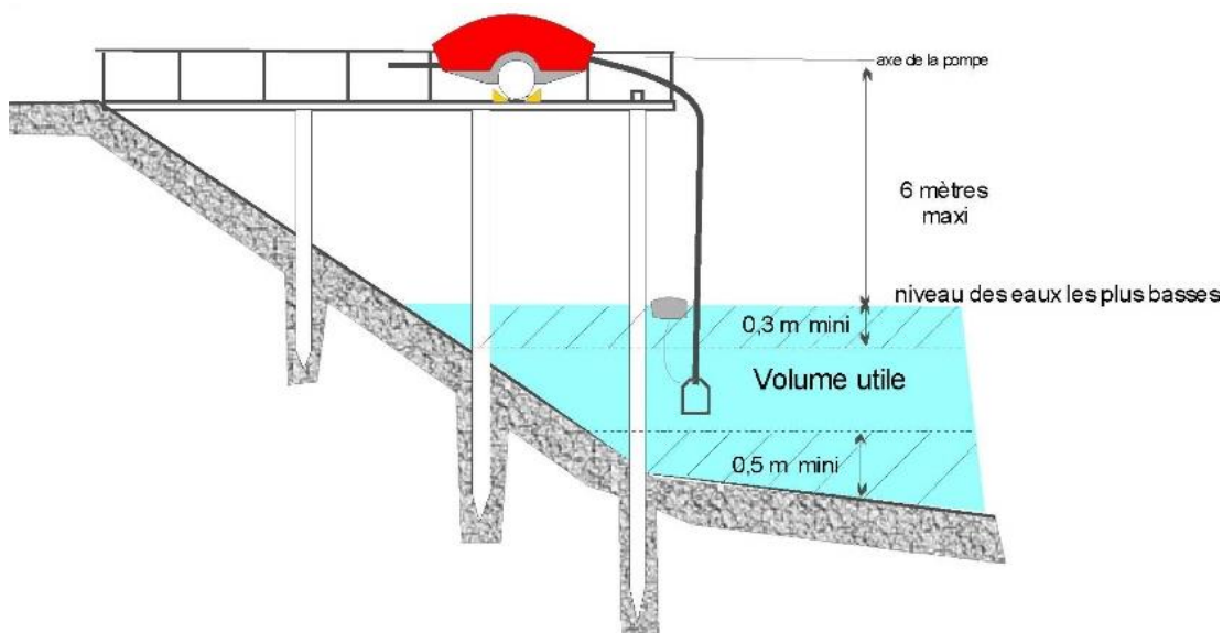
Illustration n°2 : Schéma de principe d'une estacade
