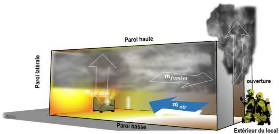
Schéma n°6 : transferts de masse
